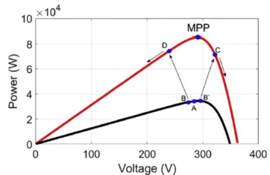
شکل (۲): مسئله راندگی در FL-MPPT
